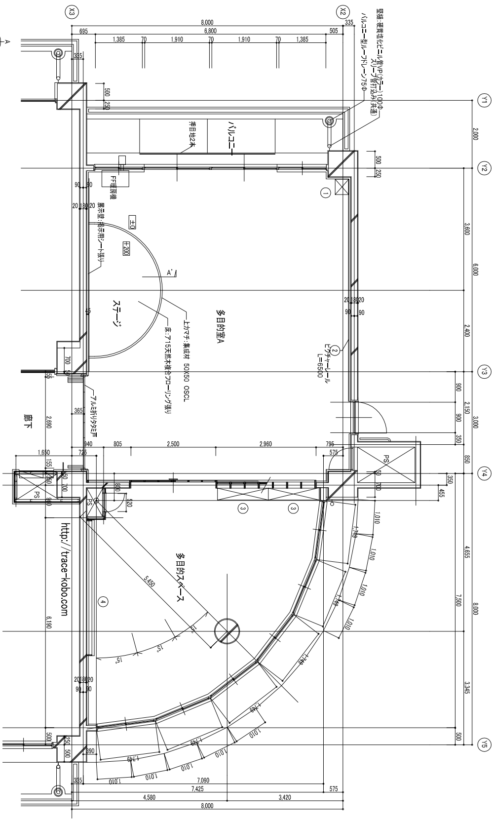
多目的スペース 平面詳細図 1/50
