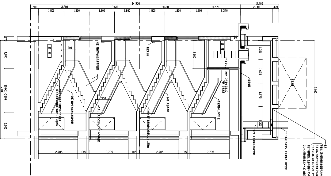
3階平面図 1:50
