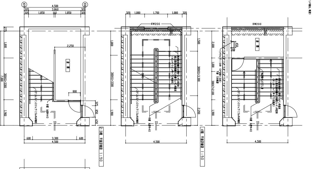
4階平面図 1:50
